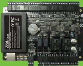
C3-200-PRO
